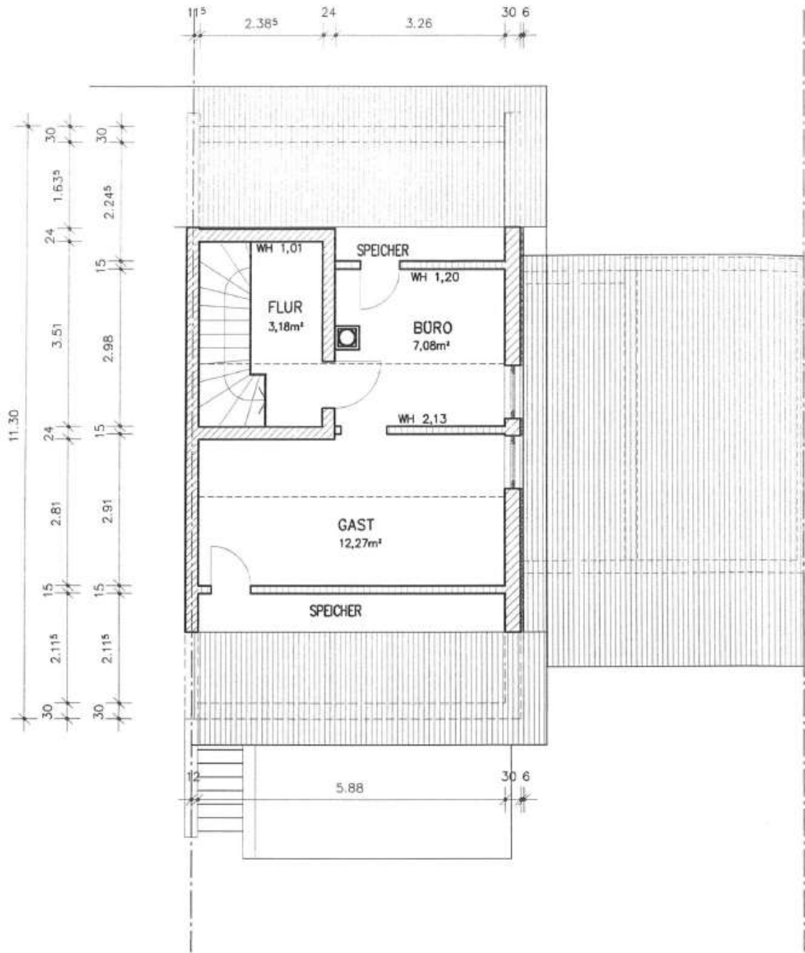
2026_DG_Bemaßter Grundriss_Tan
