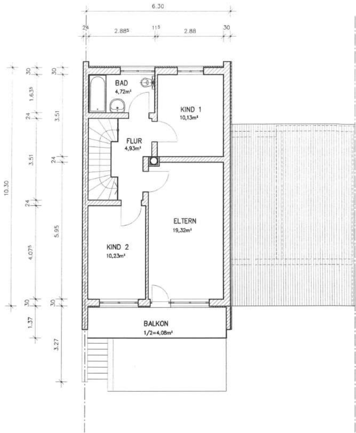
2026_OG_Bemaßter Grundriss_Tan
