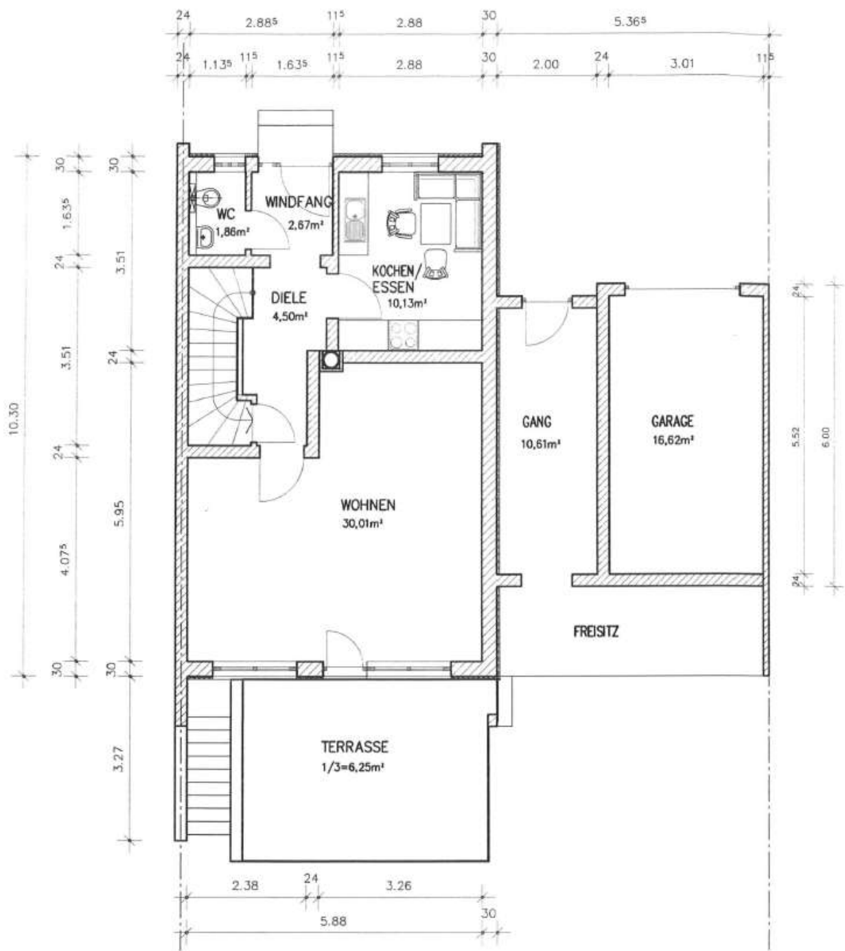
2026_EG_Bemaßter Grundriss_Tan
