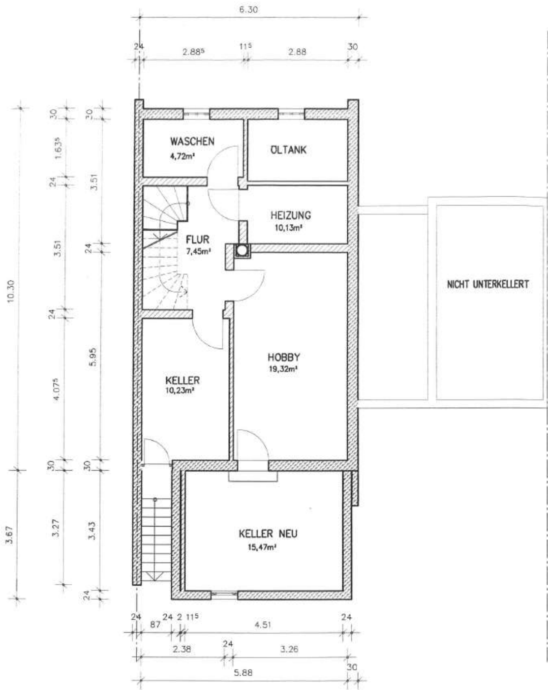
2026_KG_Bemaßter Grundriss_Tan
